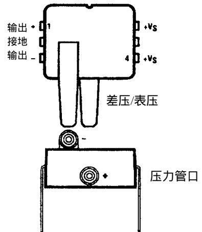
“D4”DIP(双列直插式)封装
