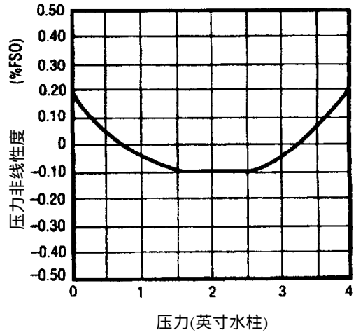
非线性度 Vs 压力
