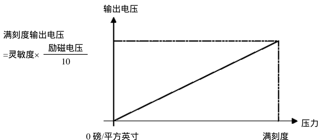
图 1 输出曲线
